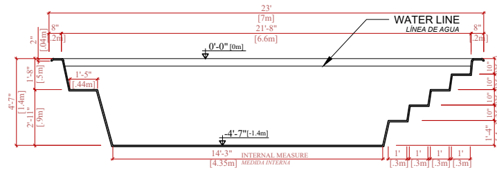
LONGITUDINAL SECTION A-A SECCIÓN LONGITUDINAL A-A
