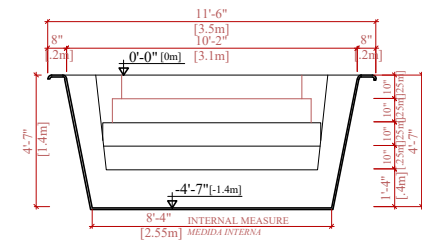
CROSS SECTION B-B SECCIÓN TRANSVERSAL B-B
