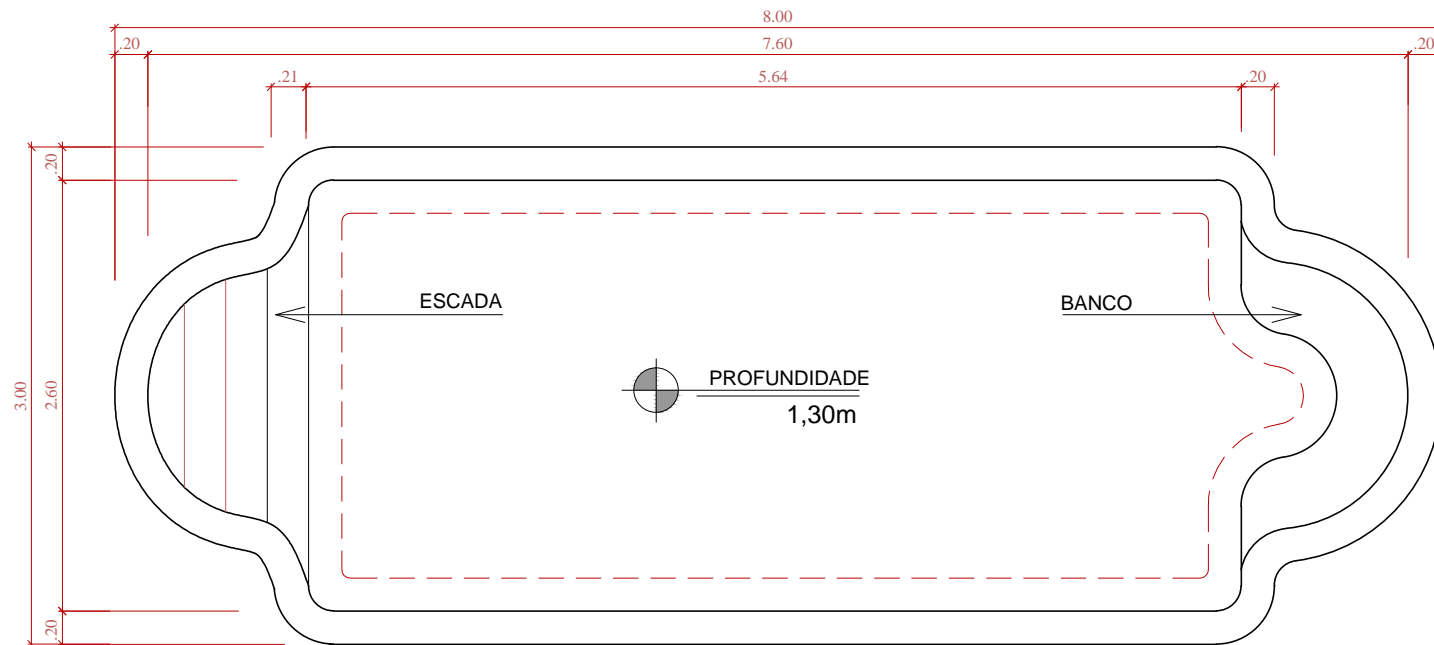
PLANTA ESCALA 1:50
