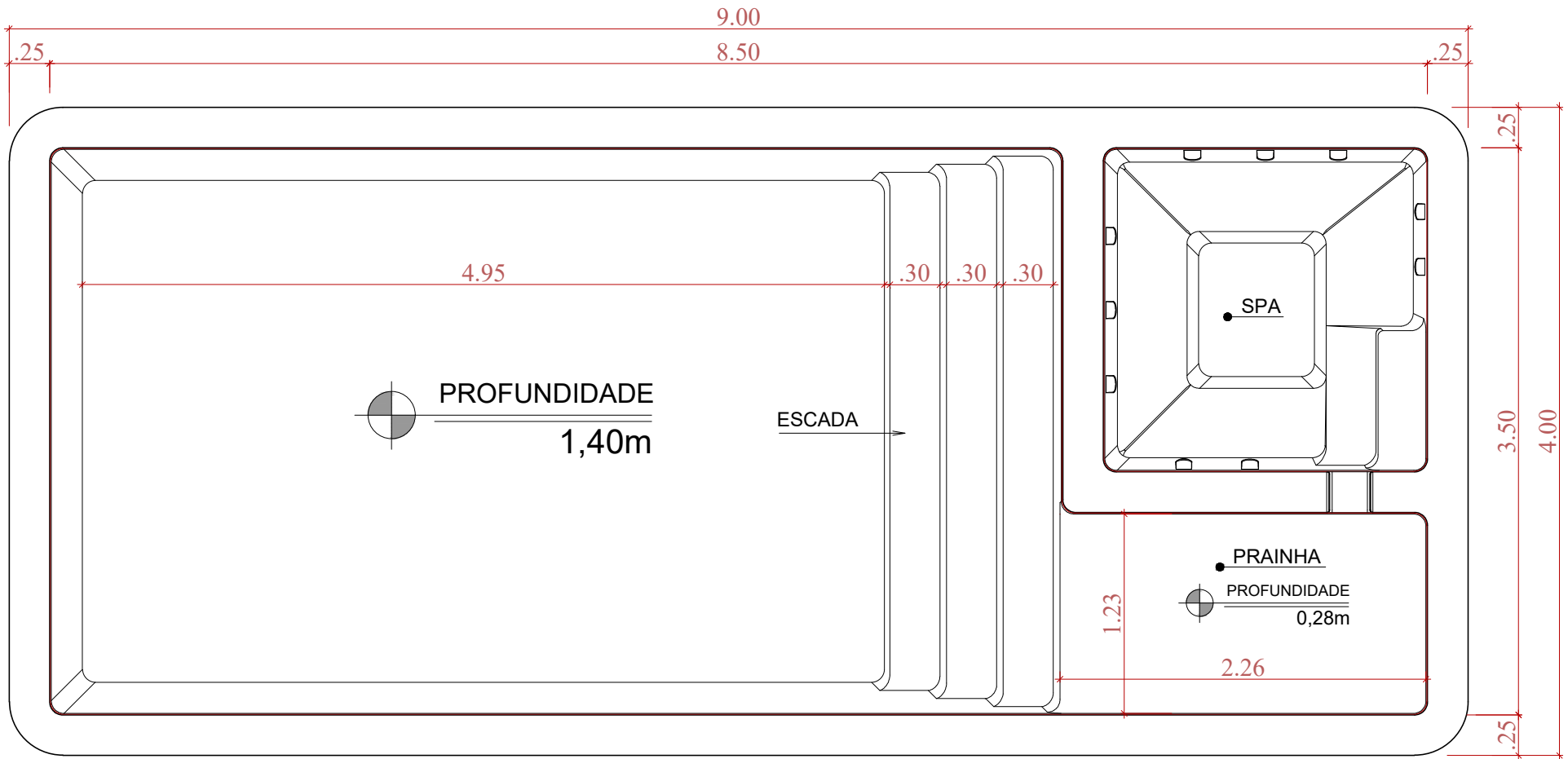
PLANTA - ATALAIA SEM ESCALA
