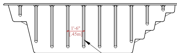
LONGITUDINAL SIDE VIEW C-C VISTA LATERAL LONGITUDINAL C-C REINFORCEMENT REFUERZO
