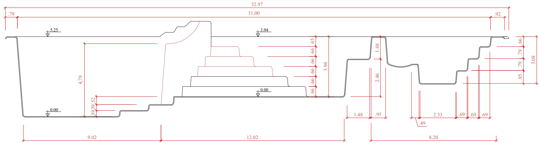
LONGITUDINAL SECTION SCALE 1:50
