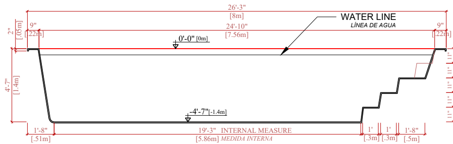
LONGITUDINAL SECTION A-A SECCIÓN LONGITUDINAL A-A
