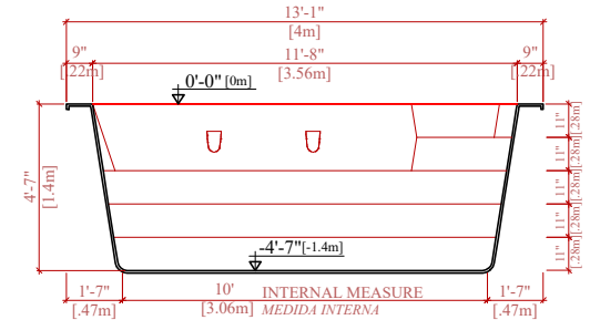
CROSS SECTION B-B SECCIÓN TRANSVERSAL B-B
