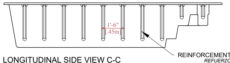
LONGITUDINAL SIDE VIEW C-C VISTA LATERAL LONGITUDINAL C-C
