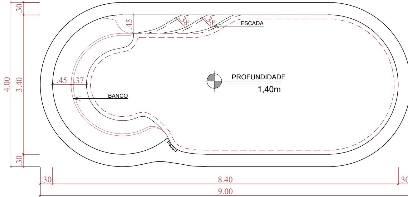
PLANTA ESCALA 1:30
