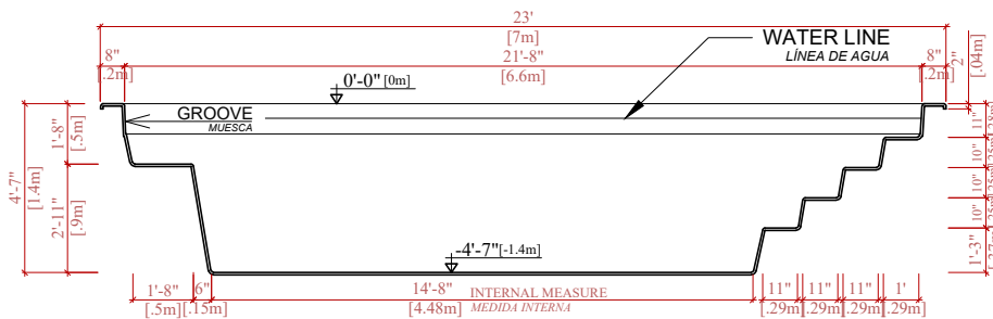
LONGITUDINAL SECTION A-A SECCIÓN LONGITUDINAL A-A
