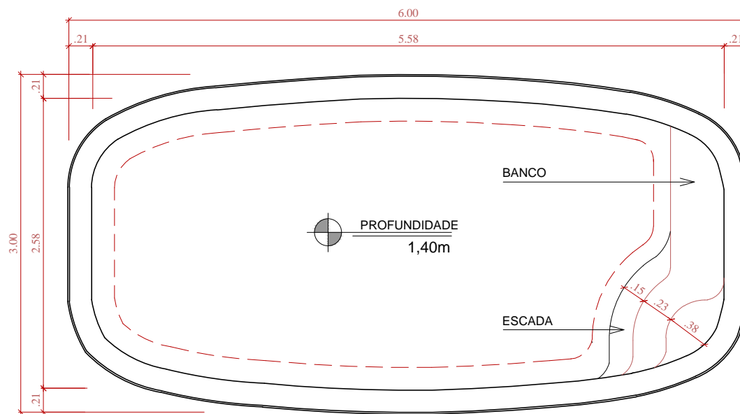
PLANTA ESCALA 1:30
