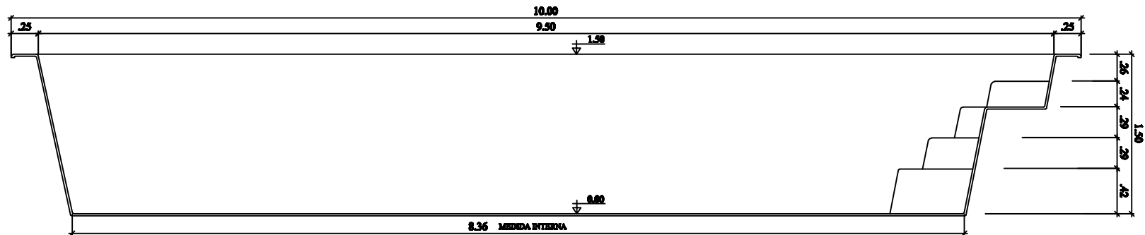
CORTE LONGITUDINAL ESCALA 1:50
