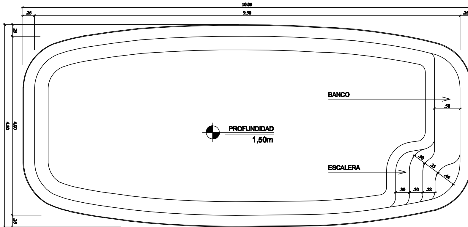
DIBUJO TÉCNICO ESCALA 1:50
