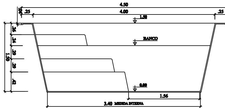
CORTE TRANSVERSAL ESCALA 1:50
