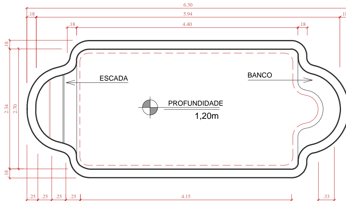
PLANTA ESCALA 1:30
