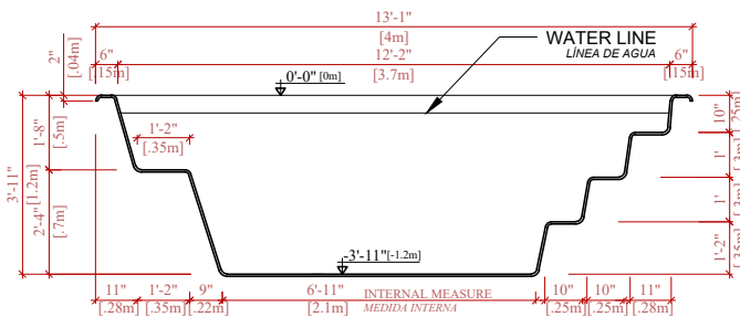
LONGITUDINAL SECTION A-A SECCIÓN LONGITUDINAL A-A
