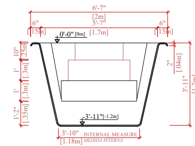
CROSS SECTION B-B SECCIÓN TRANSVERSAL B-B
