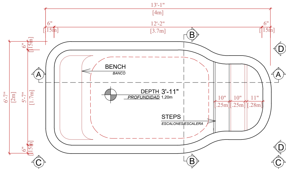
TECHNICAL DRAWING DIBUJO TÉCNICO
