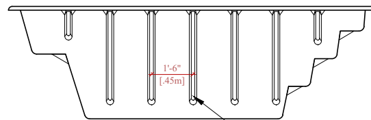
LONGITUDINAL SIDE VIEW C-C VISTA LATERAL LONGITUDINAL C-C
