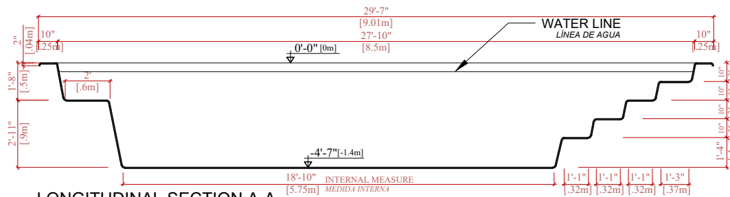
LONGITUDINAL SECTION A-A SECCIÓN LONGITUDINAL A-A
