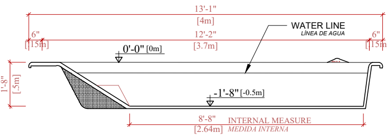
LONGITUDINAL SECTION A-A SECCIÓN LONGITUDINAL A-A
