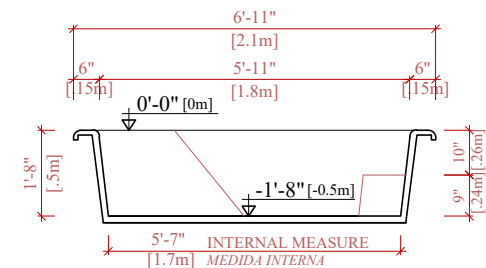
CROSS SECTION B-B SECCIÓN TRANSVERSAL B-B
