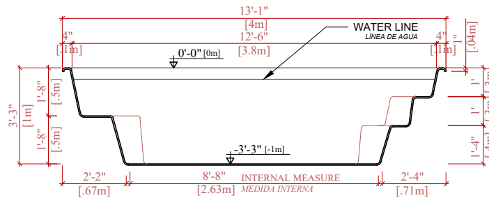
LONGITUDINAL SECTION A-A SECCIÓN LONGITUDINAL A-A
