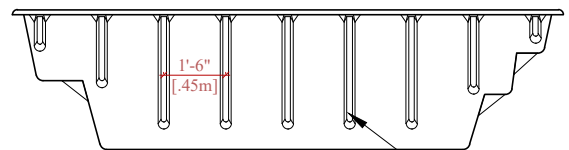
LONGITUDINAL SIDE VIEW C-C VISTA LATERAL LONGITUDINAL C-C
