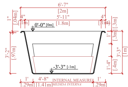
CROSS SECTION B-B SECCIÓN TRANSVERSAL B-B
