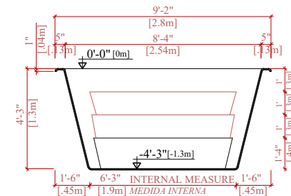
CROSS SECTION B-B SECCIÓN TRANSVERSAL B-B
