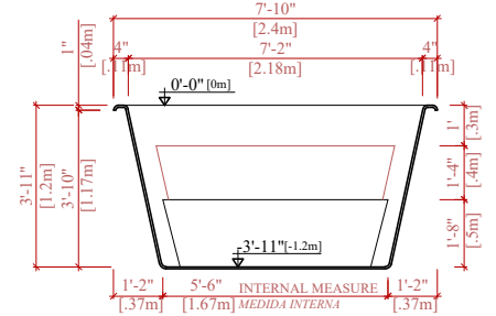
CROSS SECTION B-B SECCIÓN TRANSVERSAL B-B
