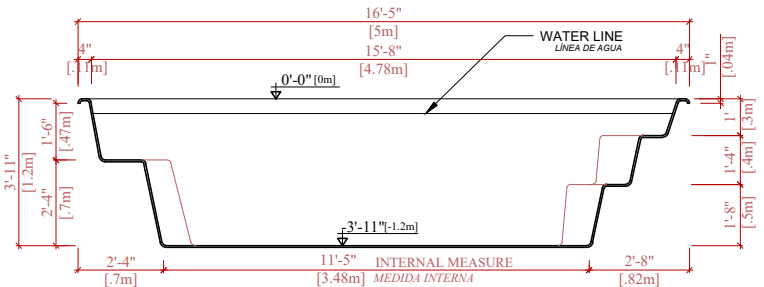
LONGITUDINAL SECTION A-A SECCIÓN LONGITUDINAL A-A
