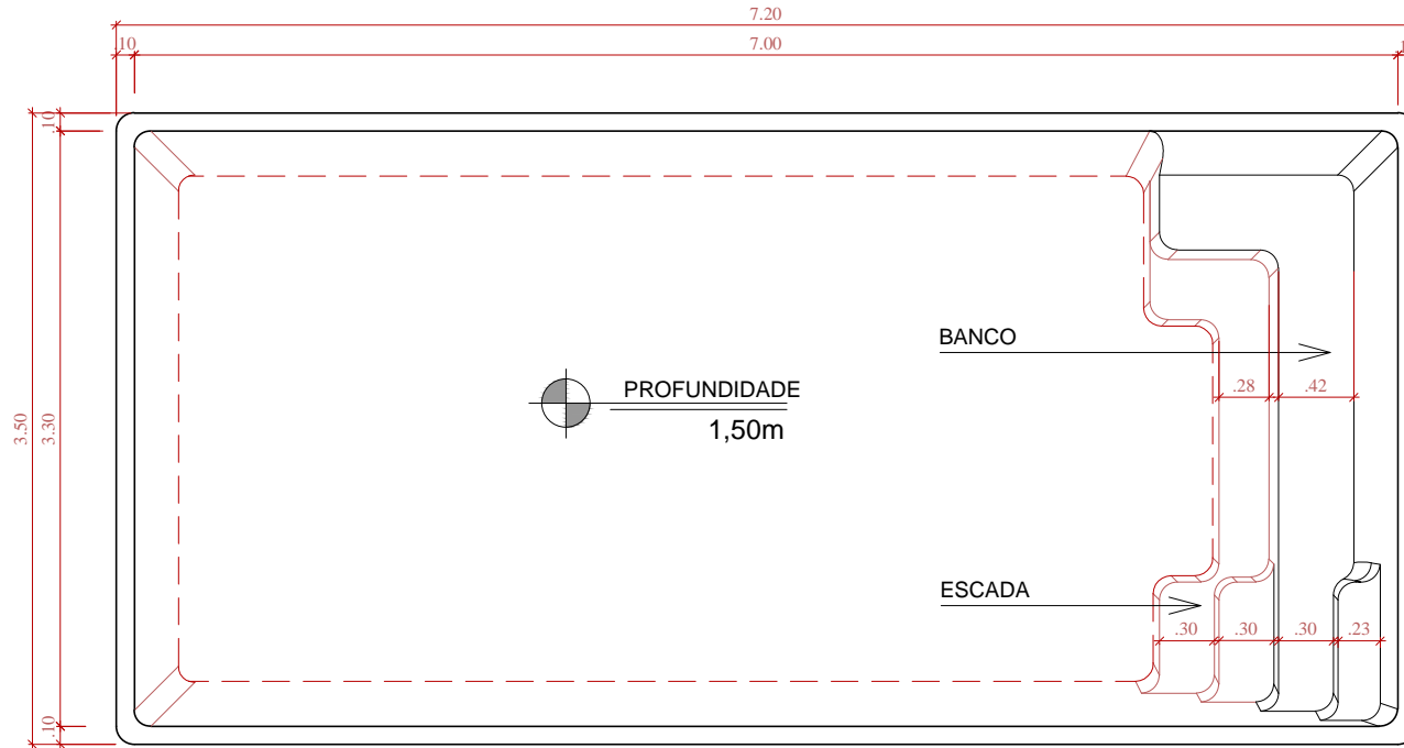
PLANTA ESCALA 1:50
