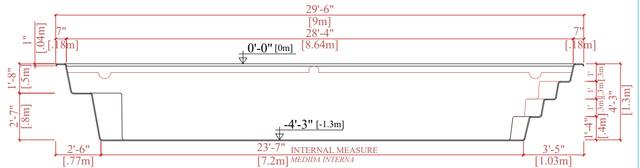
LONGITUDINAL SECTION CORTE LONGITUDINAL
