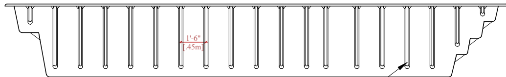
LONGITUDINAL SIDE VIEW C-C VISTA LATERAL LONGITUDINAL C-C
