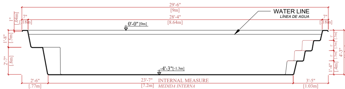
LONGITUDINAL SECTION A-A SECCIÓN LONGITUDINAL A-A
