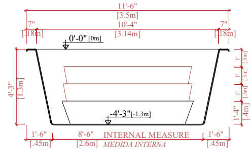
CROSS SECTION B-B SECCIÓN TRANSVERSAL B-B
