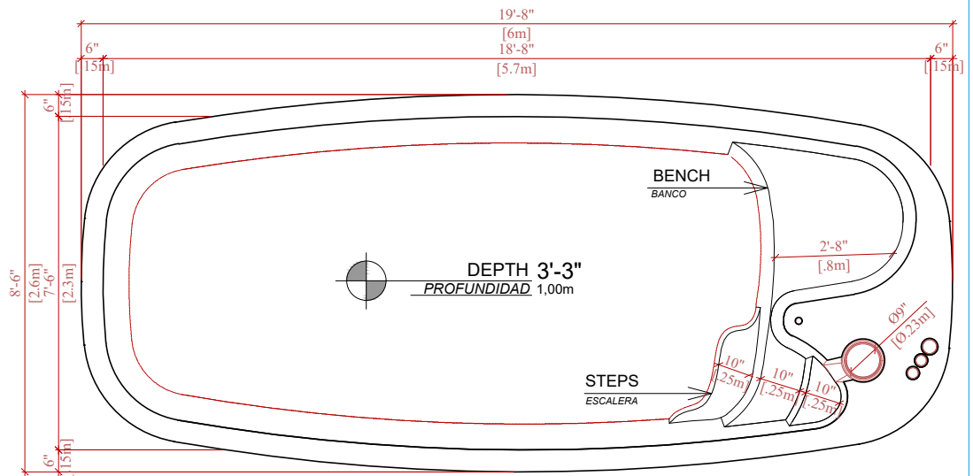
TECHNICAL DRAWING DIBUJO TÉCNICO
