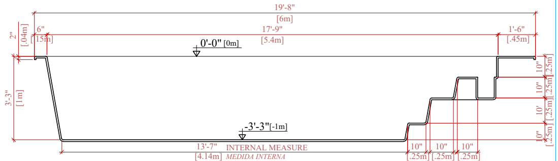
LONGITUDINAL SECTION CORTE LONGITUDINAL
