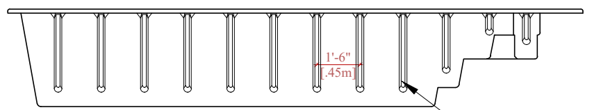
LONGITUDINAL SIDE VIEW C-C VISTA LATERAL LONGITUDINAL C-C
