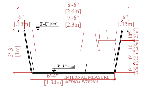
CROSS SECTION B-B SECCIÓN TRANSVERSAL B-B
