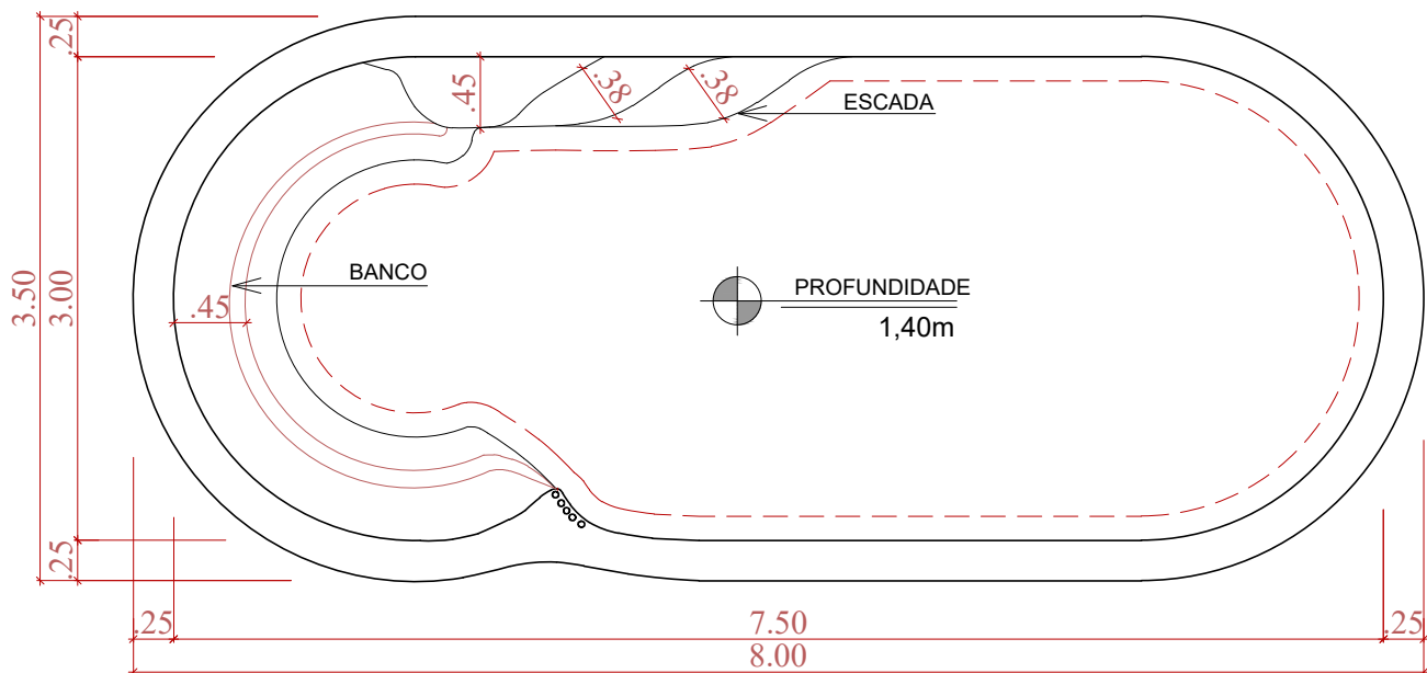
PLANTA ESCALA 1:30
