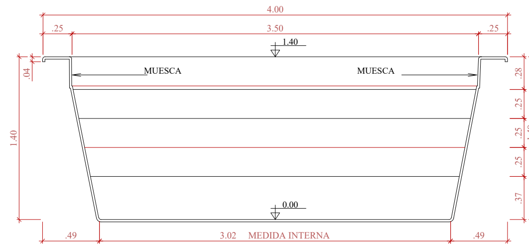
CORTE TRANSVERSAL ESCALA 1:50
