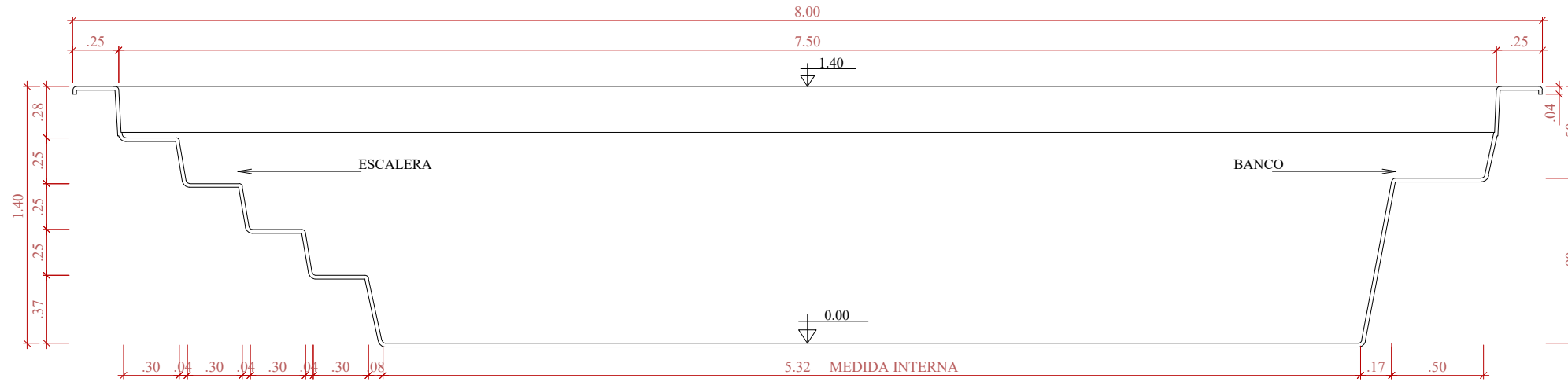
CORTE LONGITUDINAL ESCALA 1:50
