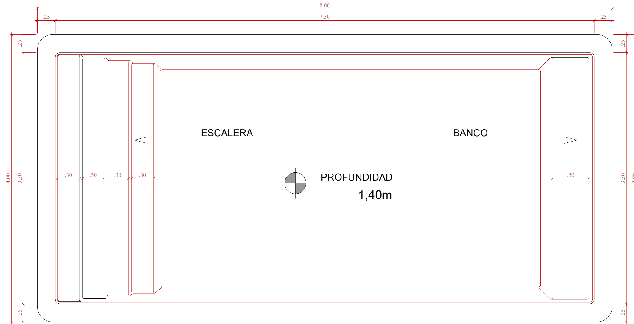
DIBUJO TÉCNICO ESCALA 1:50
