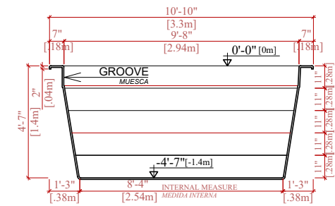
CROSS SECTION B-B SECCIÓN TRANSVERSAL B-B
