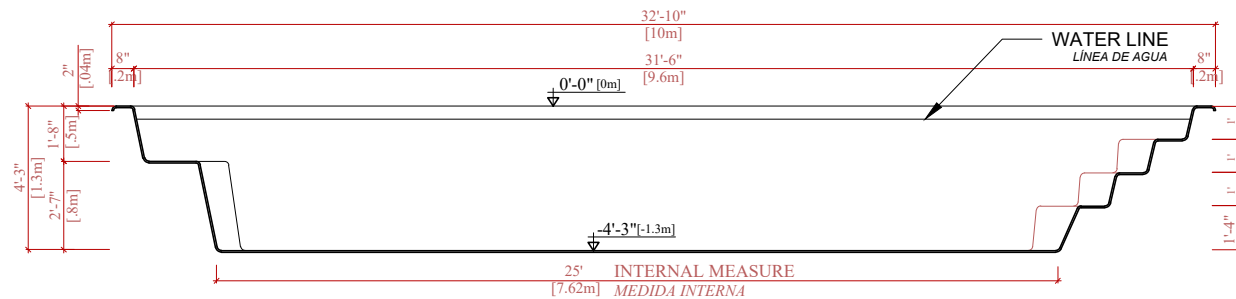
LONGITUDINAL SECTION A-A SECCIÓN LONGITUDINAL A-A
