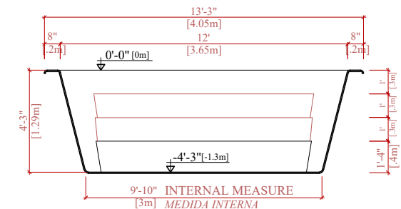
CROSS SECTION B-B SECCIÓN TRANSVERSAL B-B
