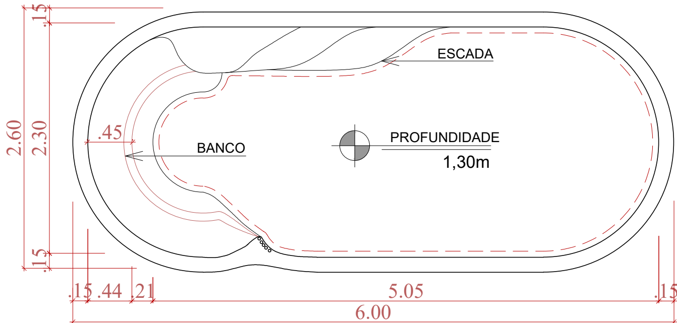
PLANTA ESCALA 1:30
