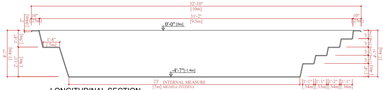
LONGITUDINAL SECTION CORTE LONGITUDINAL
