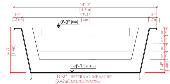
CROSS SECTION B-B SECCIÓN TRANSVERSAL B-B
