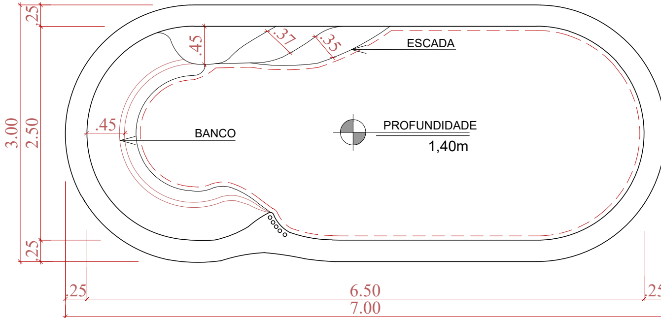
PLANTA ESCALA 1:30
