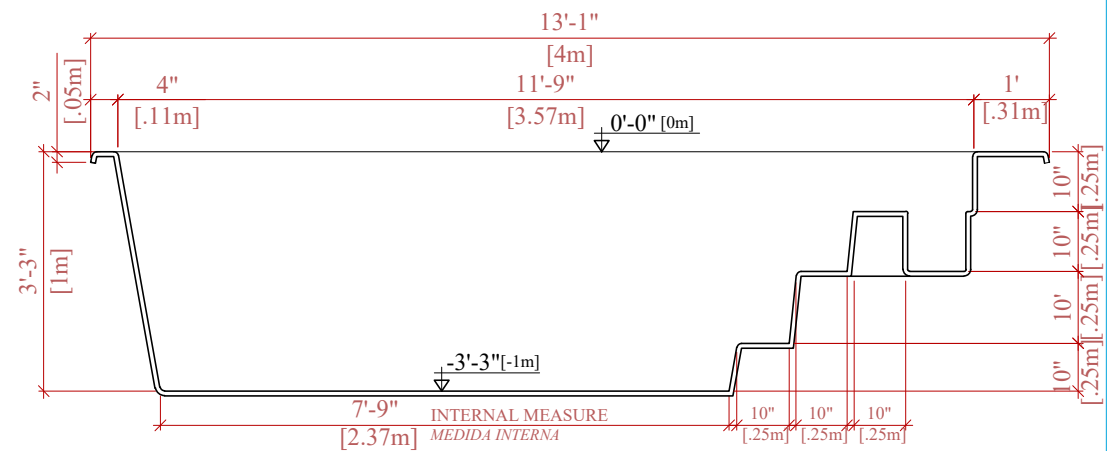
LONGITUDINAL SECTION CORTE LONGITUDINAL
