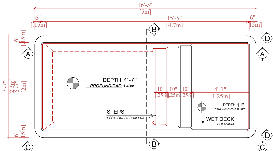
TECHNICAL DRAWING DIBUJO TÉCNICO
