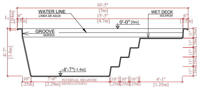
LONGITUDINAL SECTION A-A SECCIÓN LONGITUDINAL A-A
