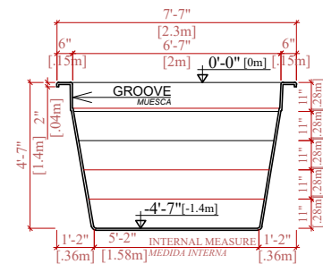
CROSS SECTION B-B SECCIÓN TRANSVERSAL B-B
